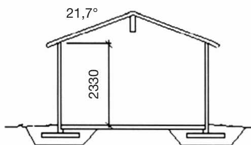
Sektion
