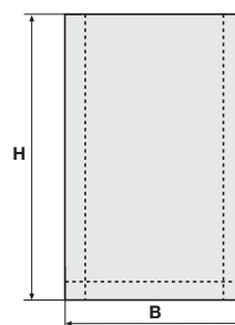
Figur 2 Pinchbotten med invikta sidor alt rak botten utan invikta sidor. I tabellerna anges måtten på produkter med invikta sidor som B/b x H. Produkter utan invikta sidor anges som B x H.
